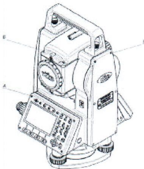
Рисунок 1 – Схема пломбирования тахеометров электронных 6Та3 от несанкционированного доступа
