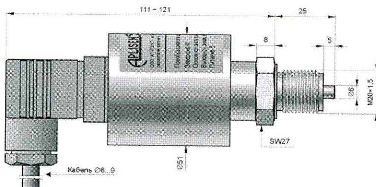
Рисунок 3 - Внешний вид, габаритные и установочные размеры преобразователей давления измерительных РС-50
