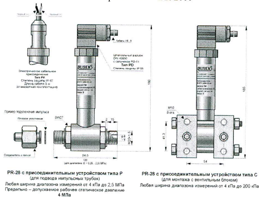
Рисунок 11 - Внешний вид, габаритные и установочные размеры преобразователей давления измерительных PR-28
