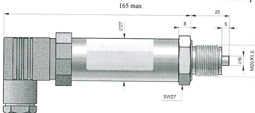
Рисунок 2 - Внешний вид, габаритные и установочные размеры преобразователей давления измерительных РС-28, РС-26Е, АРС-100Е
