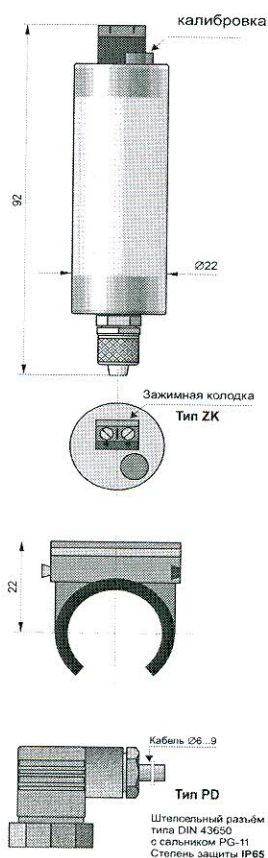
Рисунок 4 - Внешний вид, габаритные и установочные размеры преобразователей давления измерительных РС-28G
