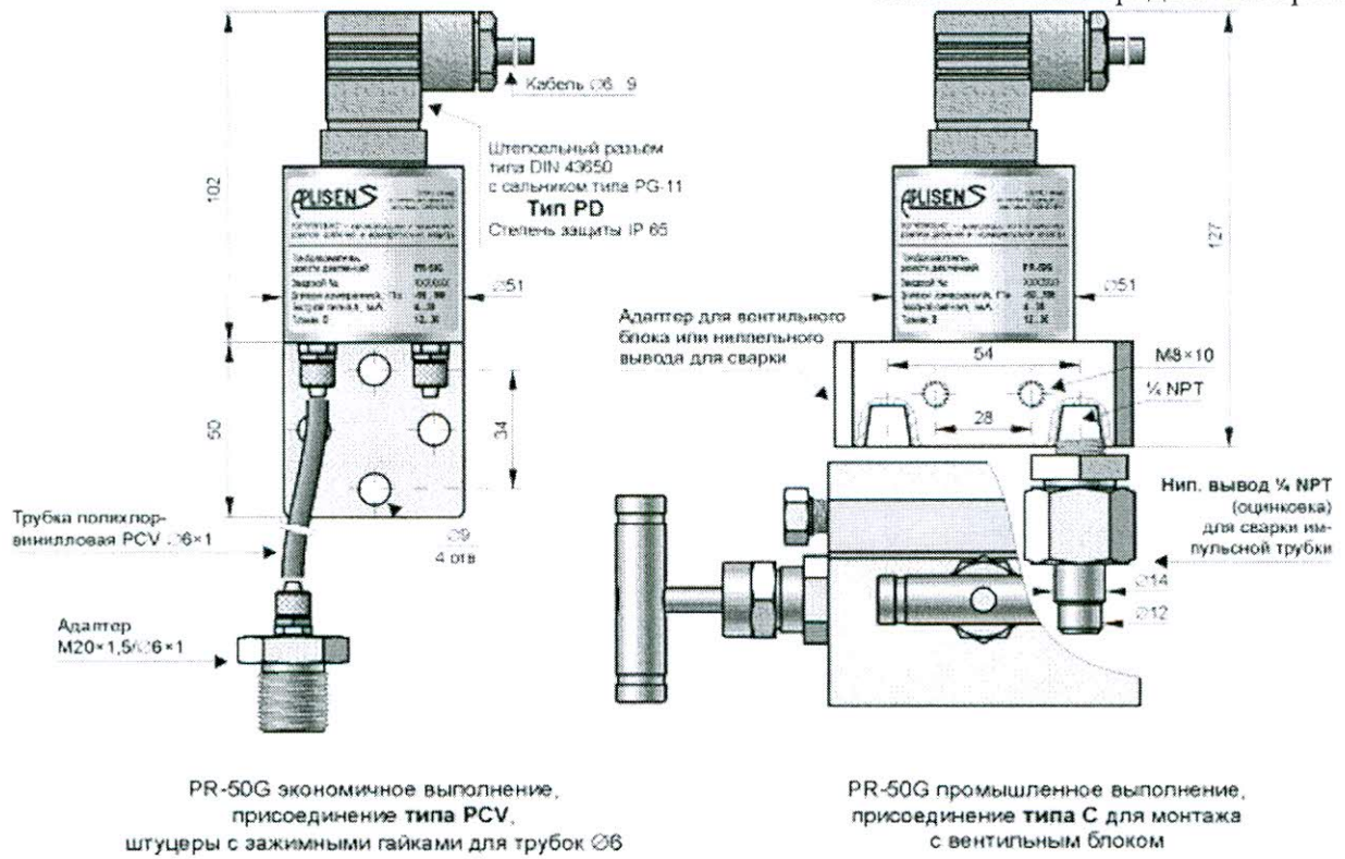
Рисунок 14 - Внешний вид, габаритные и установочные размеры преобразователей давления измерительных PR-50G
