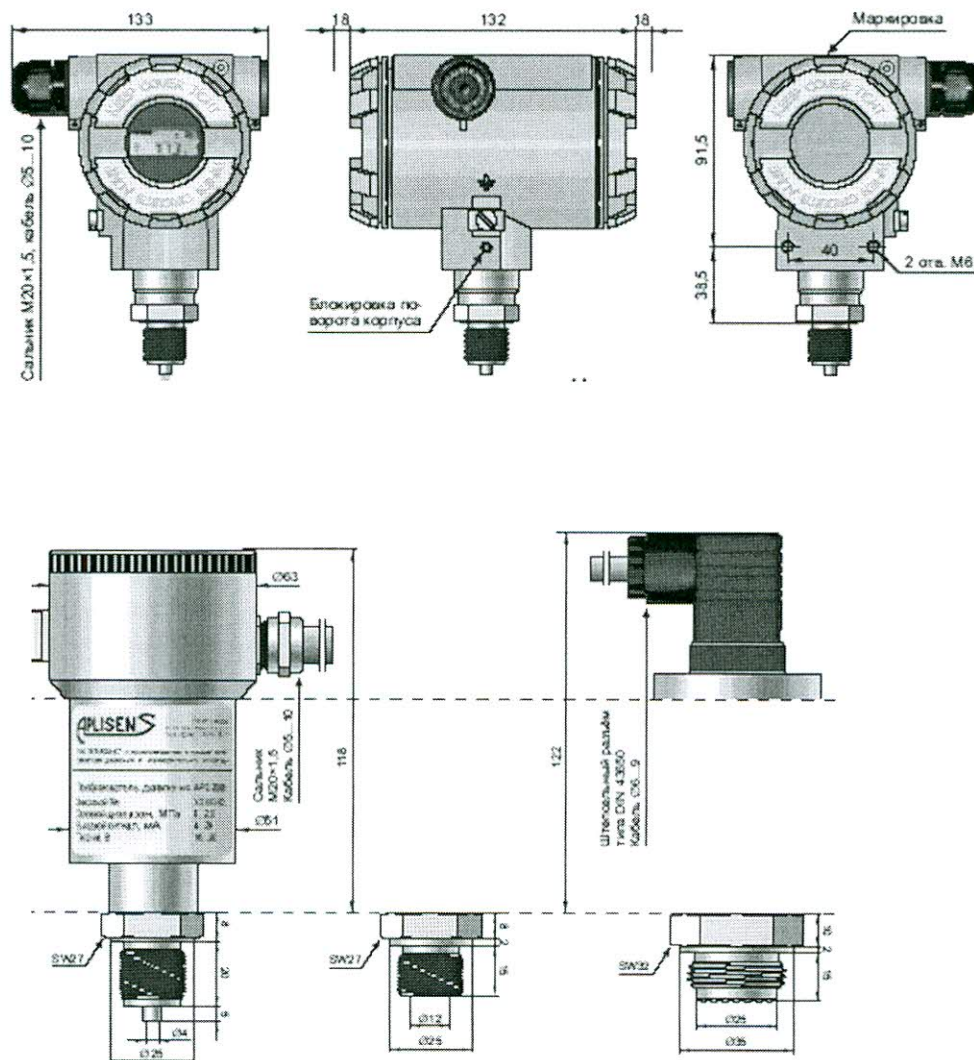
Рисунок 1 - Внешний вид, габаритные и установочные размеры преобразователей давления измерительных APC-2000
