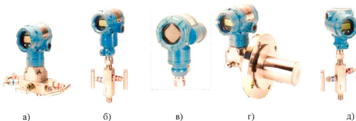
Рисунок 1 – Преобразователи давления измерительные 2051:
