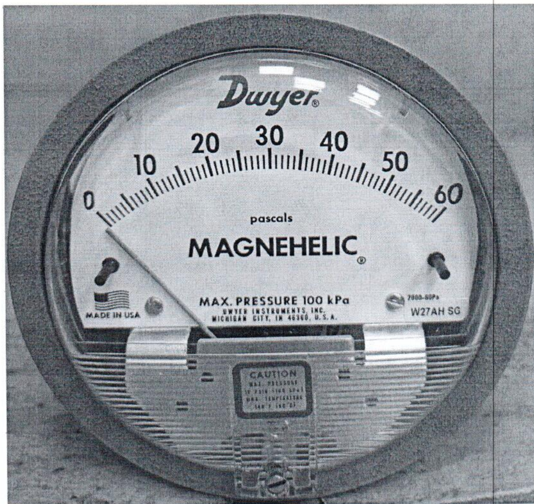
Рисунок 1.1 – Фотография общего вида манометра дифференциального показывающего Magnehelic 2000-60РА № 161222СК-10
