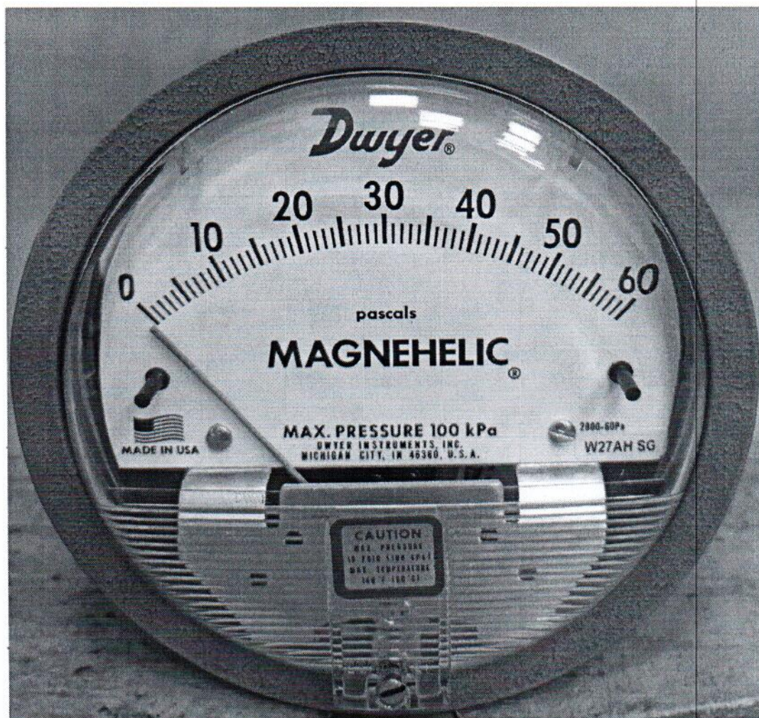
Рисунок 1.1 – Фотография общего вида манометра дифференциального показывающего Magnehelic 2000-60PA № 161222СК-39
