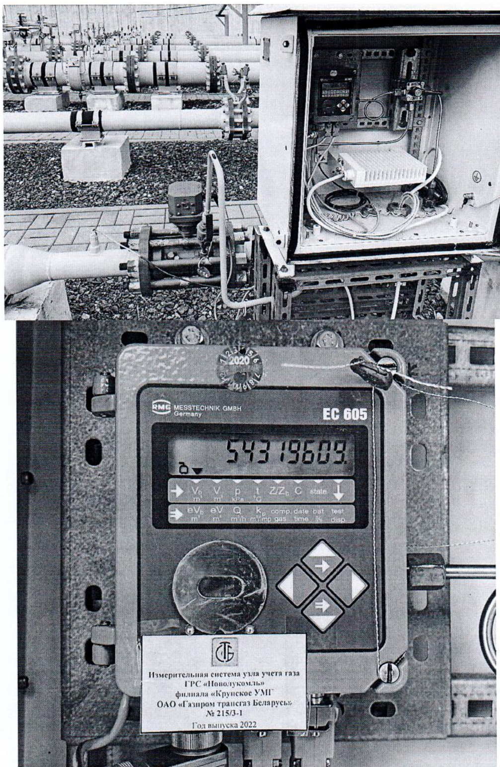
Рисунок 1.1 – Фотография общего вида ИС УУГ
