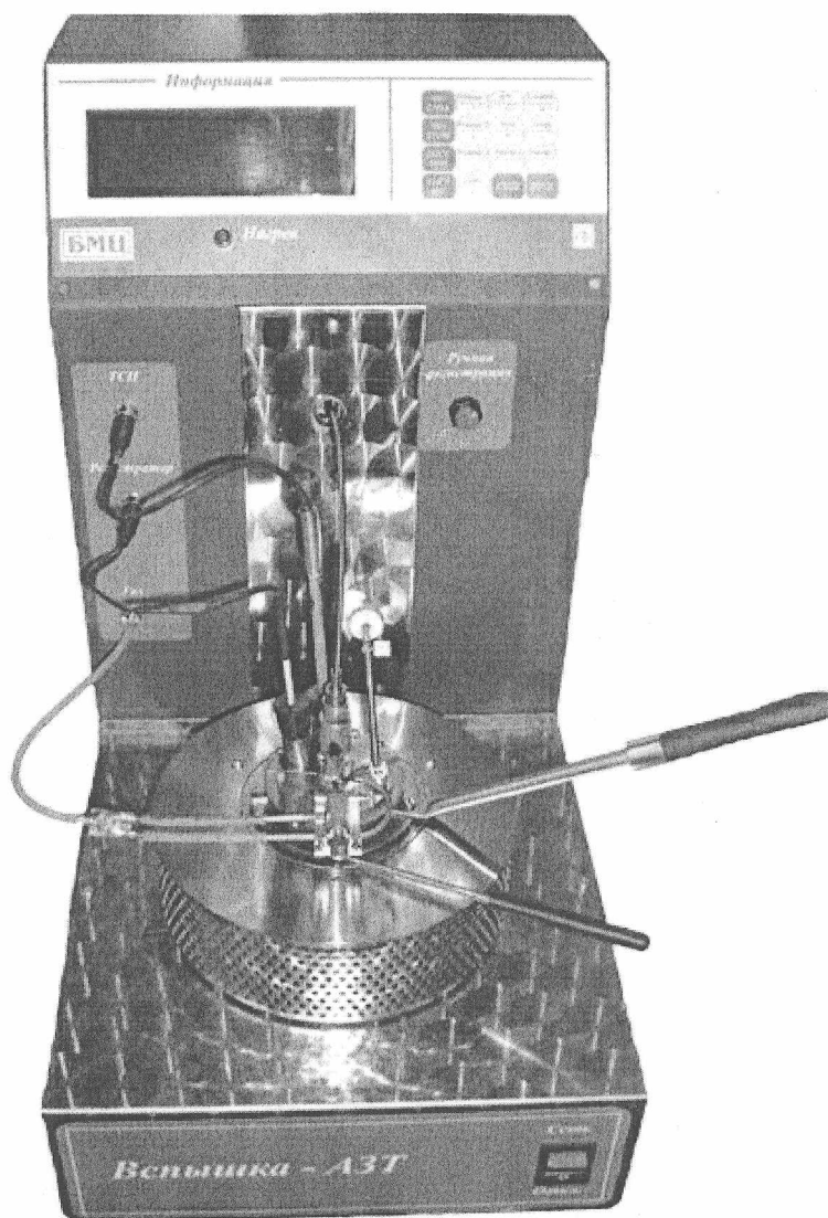
Рис. 1 Внешний вид регистратора «Вспышка-АЗТ»
