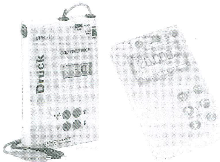
Рисунок 2. Внешний вид калибраторов UPS II, UPS III.
