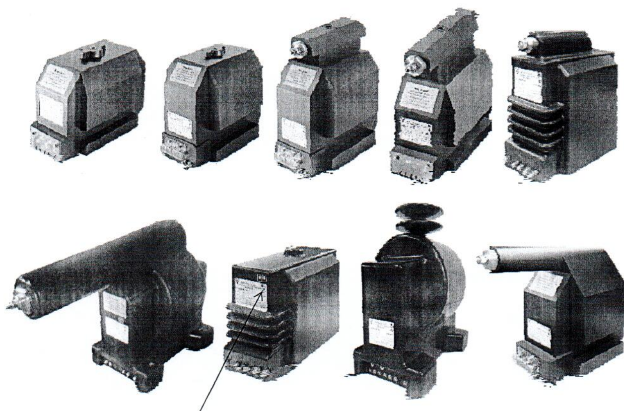
Рисунок 3 – Общий вид трансформаторов напряжения внутренней установки
